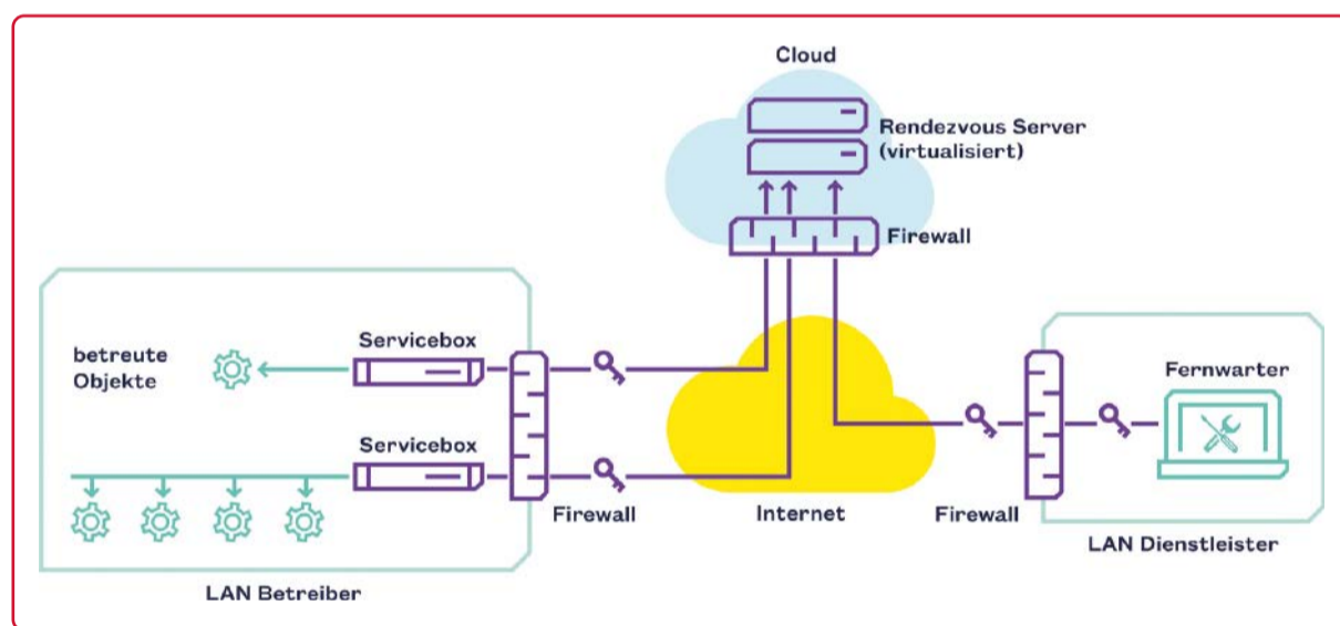
Bei der Rendezvous-Lösung von Genua werden keine einseitigen Zugriffe vom Fernhaltungsservice in Kundennetze zugelassen. Stattdessen laufen alle Wartungsverbindungen über einen Rendezvous-Server z.B. in einer demilitarisierten Zone (DMZ) oder einer Cloud.
