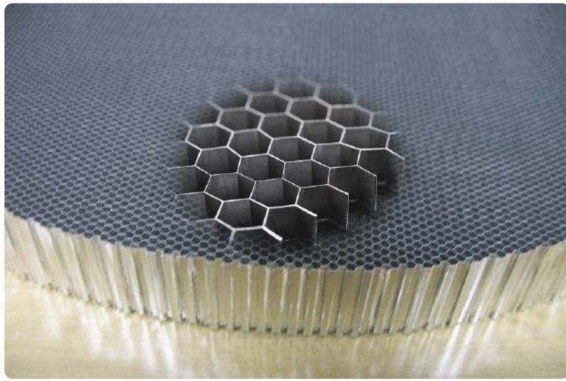
Wabenkörper aus Aluminium, der mit dem Katalysator Formalpure beschichtet wurde.
