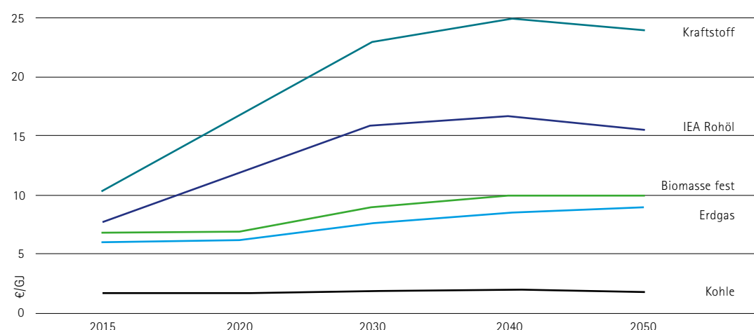
Preisentwicklung Energieträger (eigene Darstellung, WEO 2016, BCG, Prognos)
